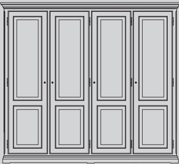
RU-108E Schrank 4 trg. Innen: Li: 1 Fachboden, 1 Stange Re: (1 trg.) 4 Fachböden H/B/T: 215 x 240 x 62
